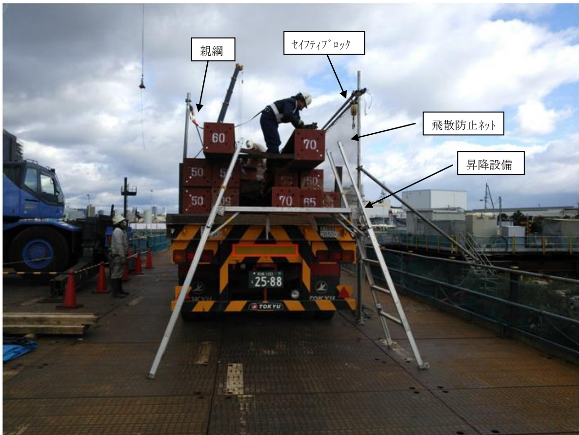
写真 1 親網及びセーフティブロック、設置状況、昇降設備、小物の落下による飛散防止ネットの設置及び使用状況
